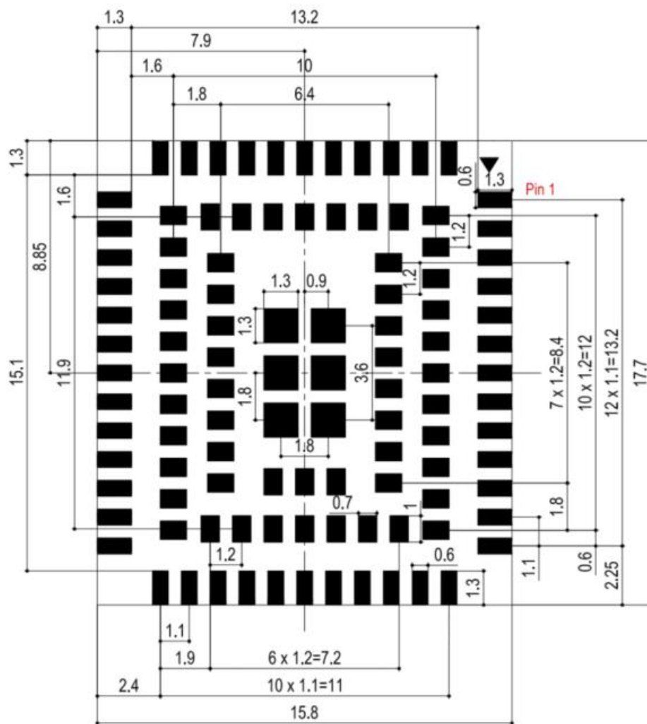
GM07 模块底视图(单位: mm)
