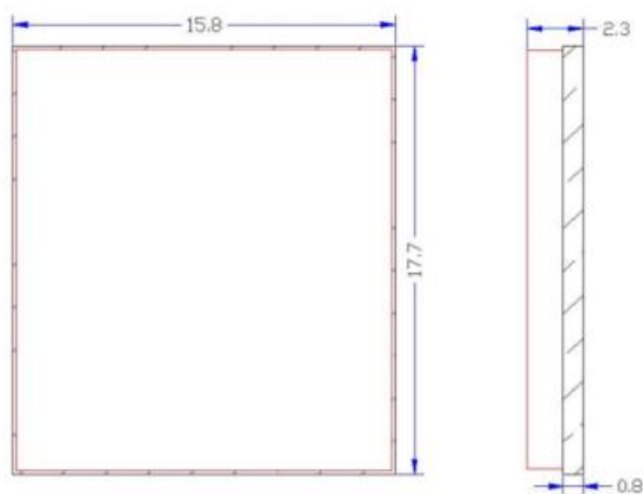
GM07 模块正视图与侧视图(单位: mm)
