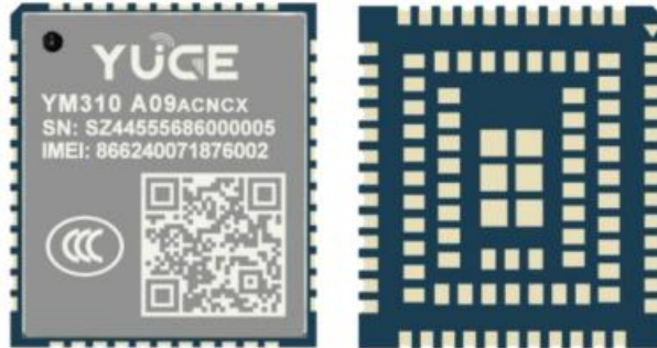
GM07（域格 YM310 A09）模块实物图(单位:mm)
